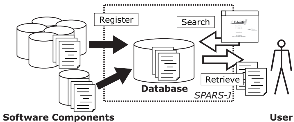
図 1.1: SPARS-J
