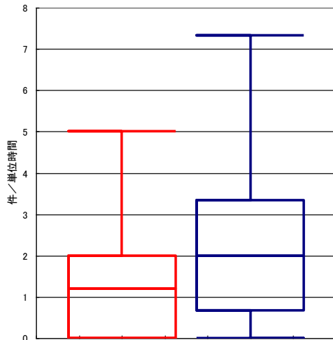
図 12 改善前後の単位時間単位指摘件数の箱ひげ図
