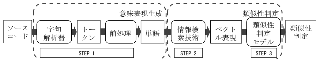
図 3.2 調査に用いるコード片類似性判定法の概要
