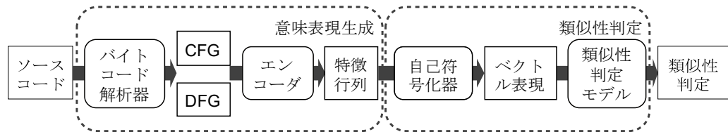
図 3.1 DeepSim の概要
